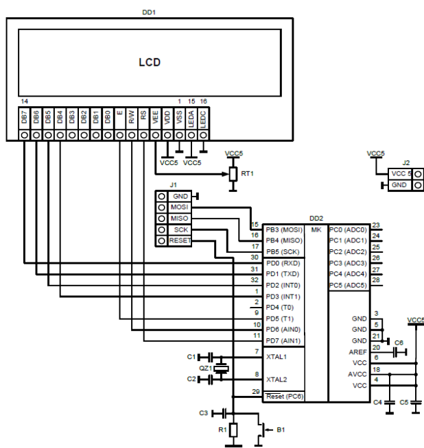
Рисунок 2 Схема электрическая принципиальная разрабатываемого устройства
