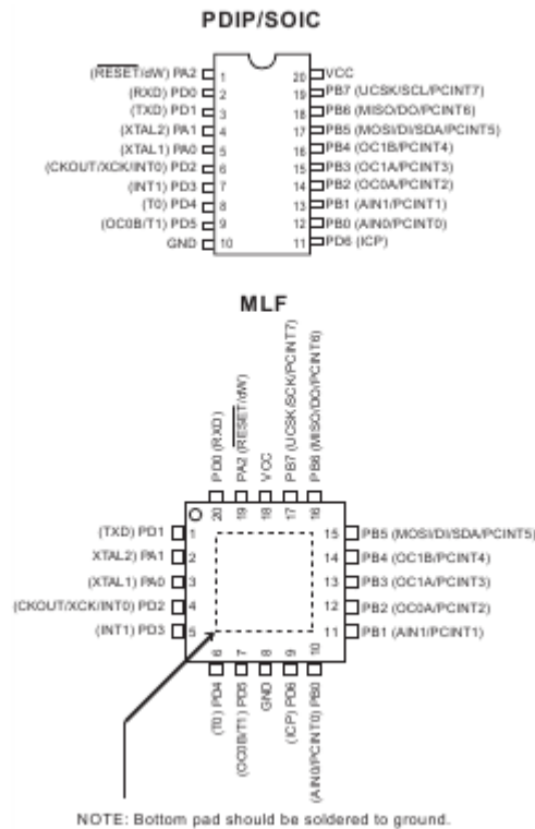
Рисунок 1. Расположение выводов (вид сверху) микроконтроллера ATtiny2313 для вариантов исполнения PDIP, SOIC и MLF
